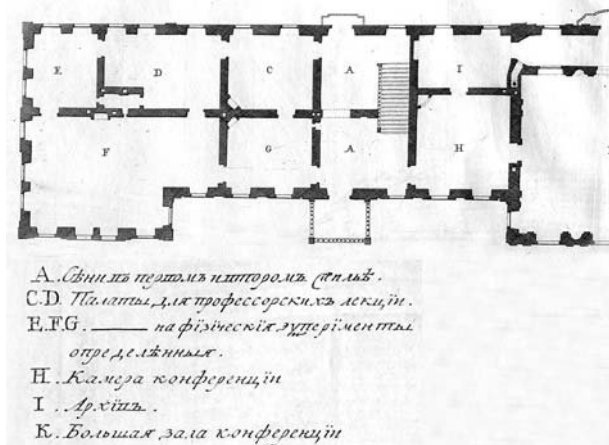
Рис. 3. План Императорской Академии наук (Дворец Прасковьи Федоровны). 2 этаж, западное (левое) крыло. 1741 г. (СПФ АРАН. Р. VI. Оп. 1. Д. 697/П-22. Л. 6 об.)
