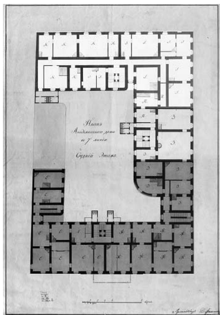
Рис. 7. Дом Академиков. План архитектора Д. Е. Филиппова. Средний этаж (СПФ АРАН. Ф. 4. Оп. 22. Д. 56. Л. 2)
