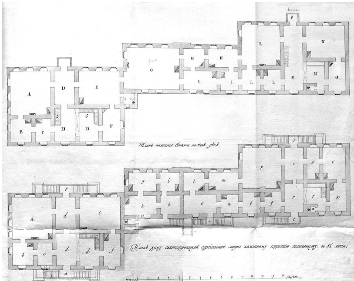
Рис. 6. План дома Троице-Сергиевой лавры на углу Большой Невы и 15-й линии (СПФ АРАН. Ф. 3. Оп. 1. Д. 219. Л. 200)
